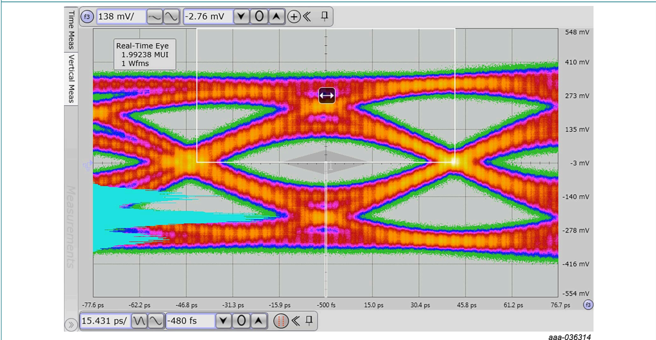
Worst cable model (WCM3), 6dB
