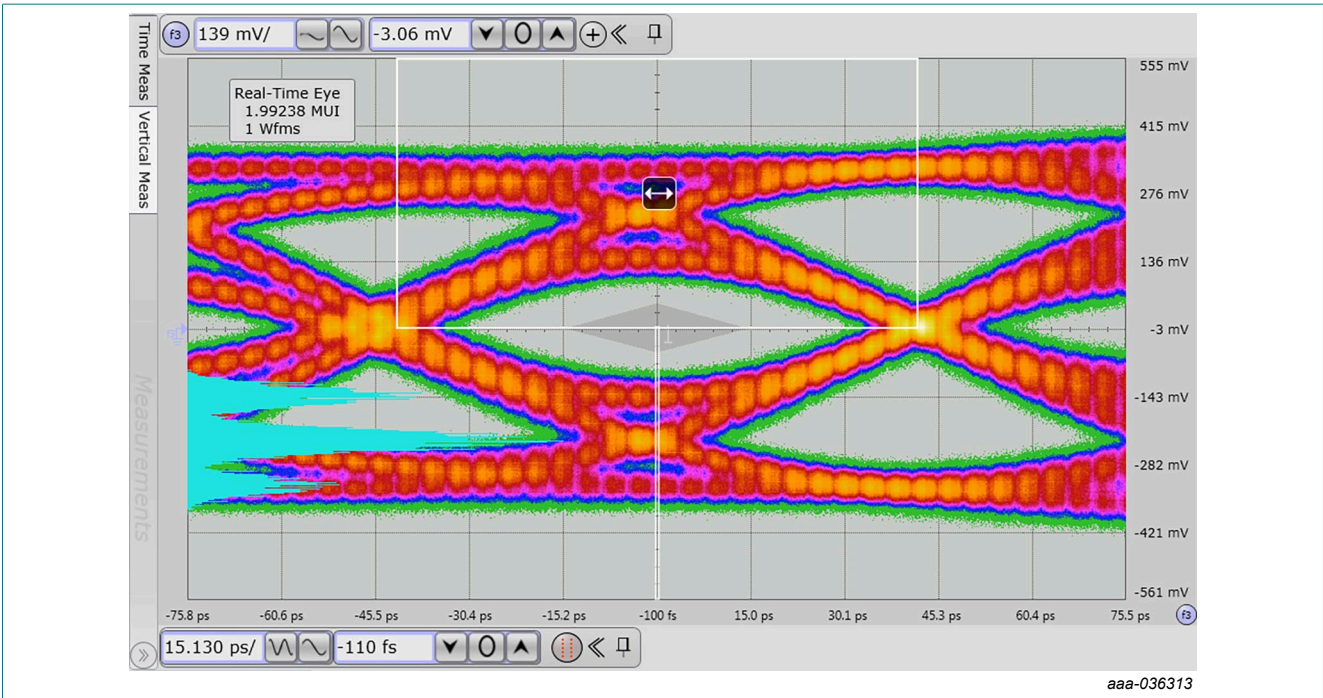
Worst cable model (WCM3), 7dB
